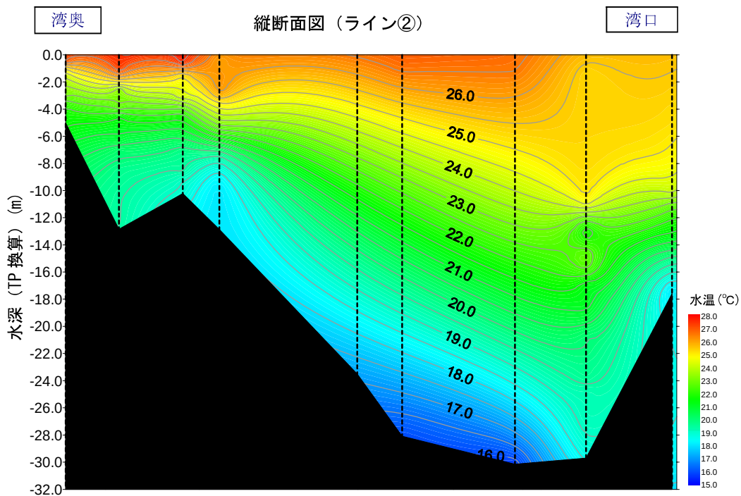
図 2-2：縦断面図（ライン②）
