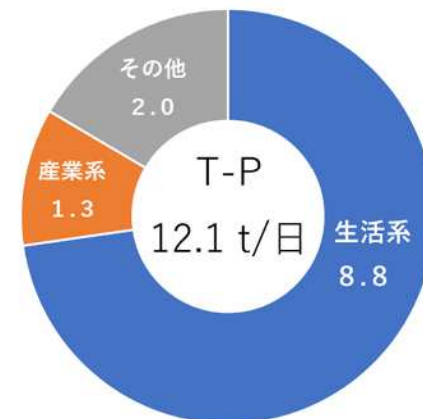
りん含有量(T-P)
