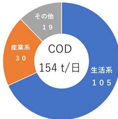
化学的酸素要求量(COD)
