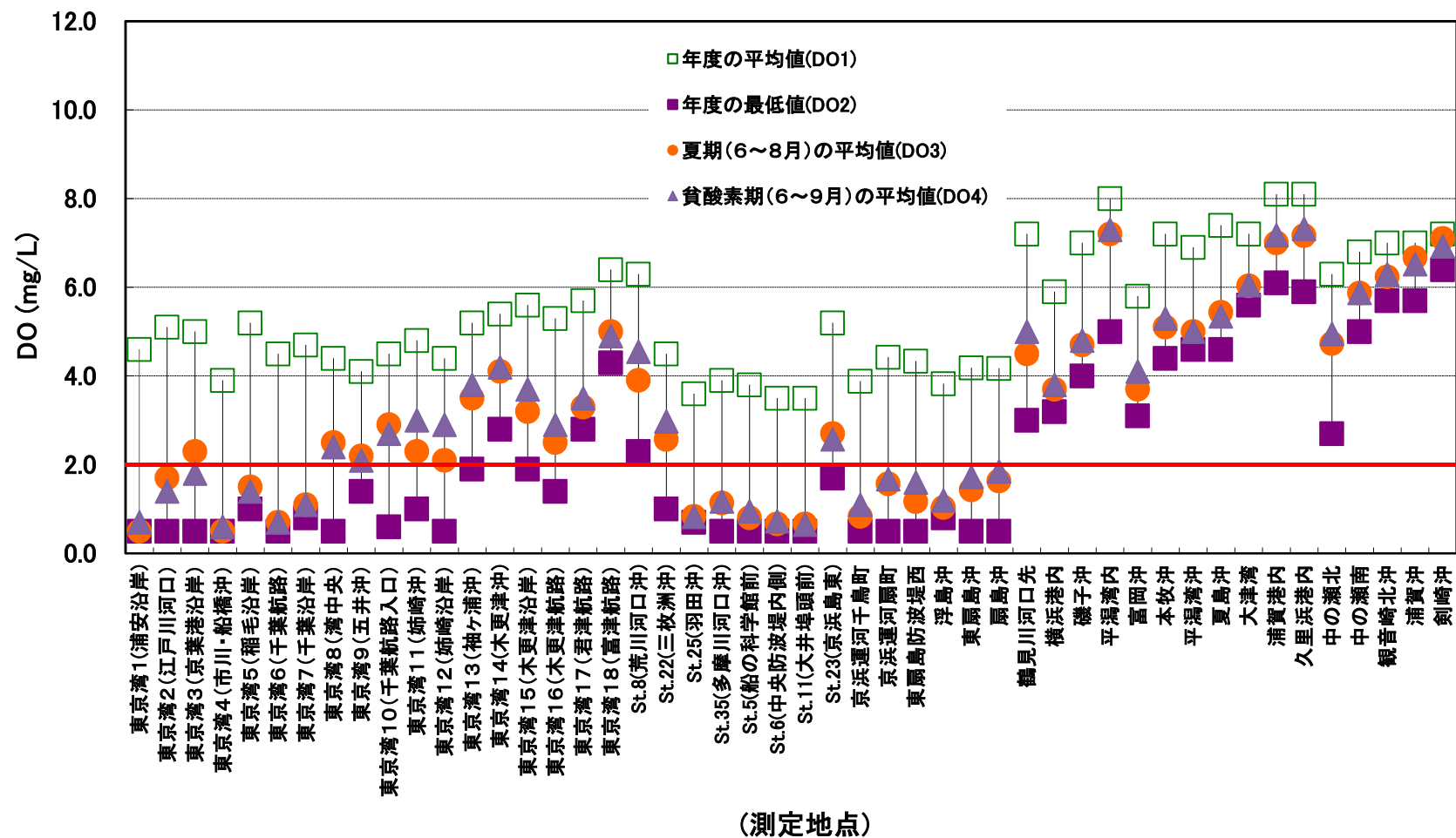
図14 令和元年度底層水の溶存酸素量調査結果
