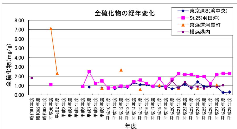
図12 COD、全りん、全硫化物の経年変化
