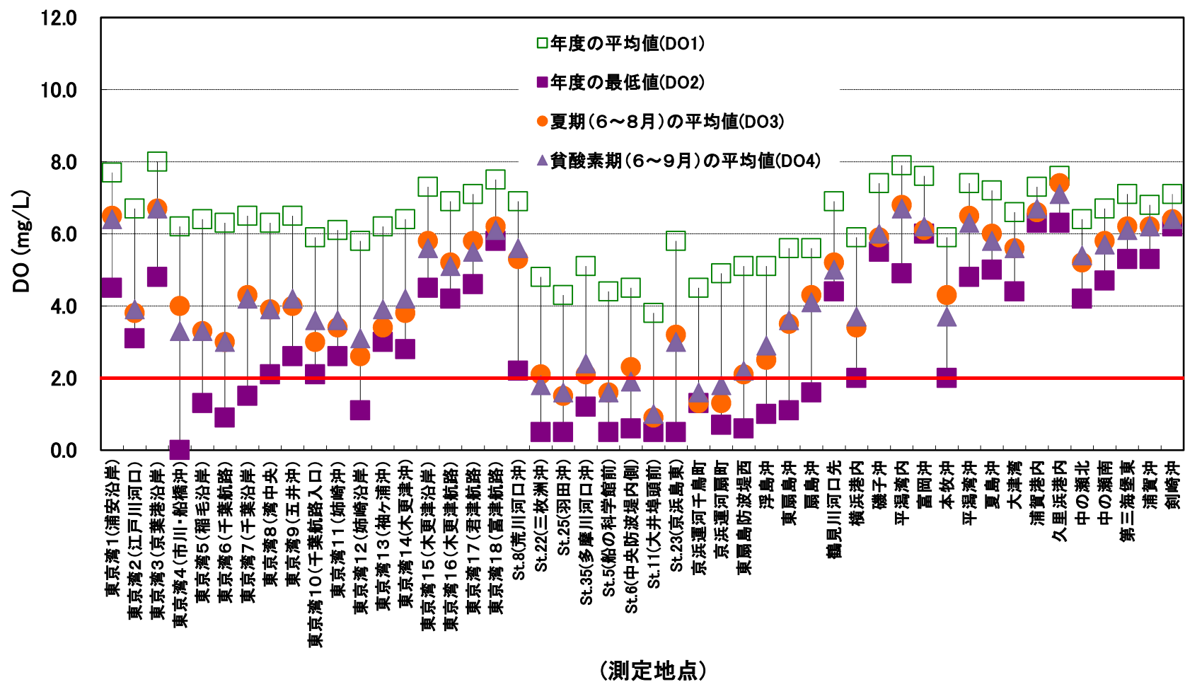
図14 平成29年度底層水の溶存酸素量調査結果
