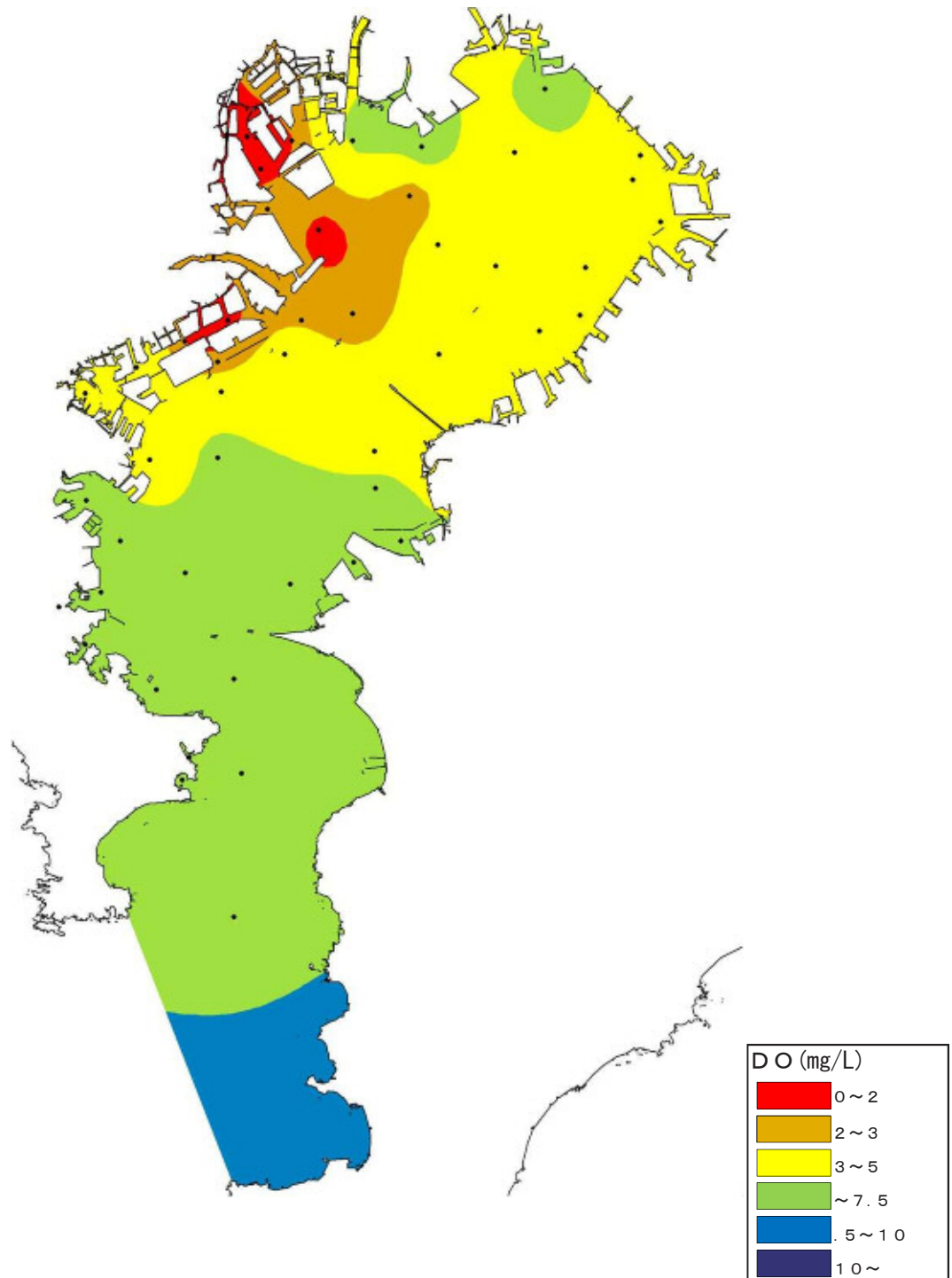
図15-2 底層D0の分布 （全48地点）
