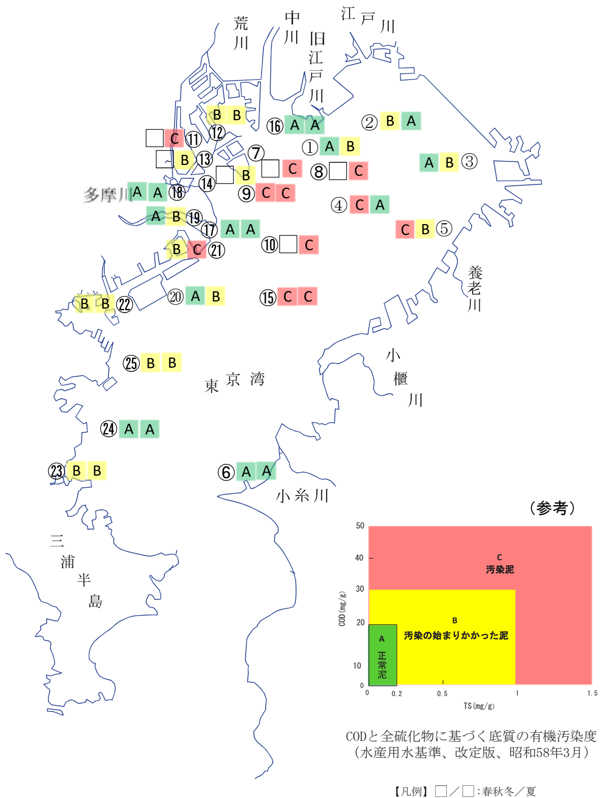
図5 有機汚染度 (全25地点)
