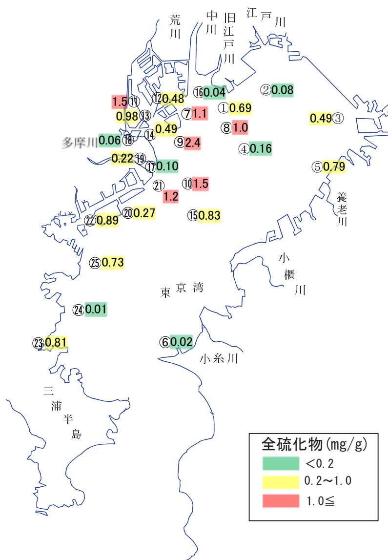
図10 全硫化物の分布 (単位 mg/g、全25地点)
